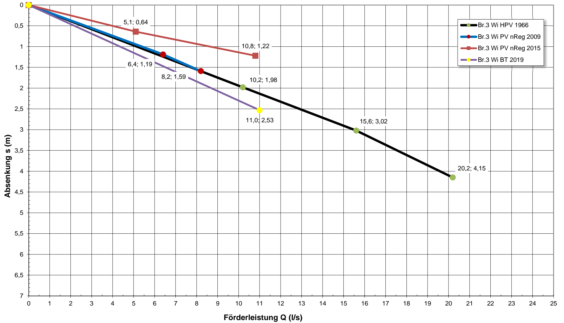
Q-s Diagramm: Brunnen 3 WSG Wintersdorf
