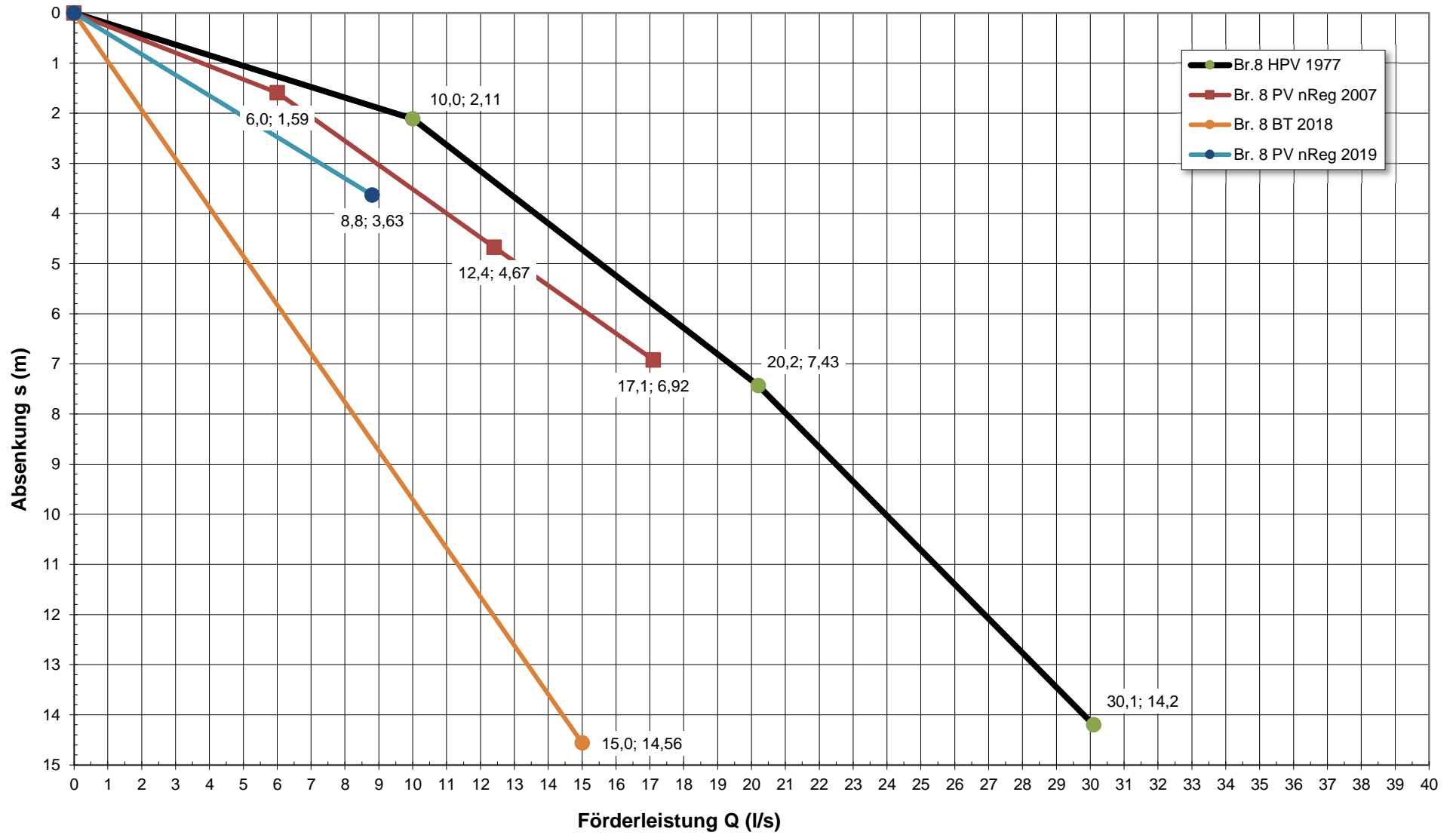
Q-s Diagramm: Brunnen 8 WSG Wintersdorf
