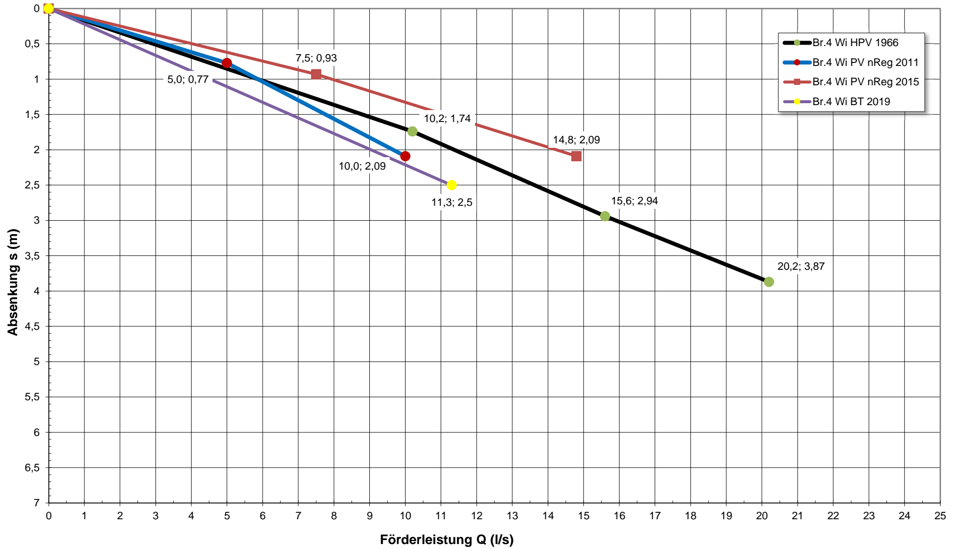
Q-s Diagramm: Brunnen 4 WSG Wintersdorf
