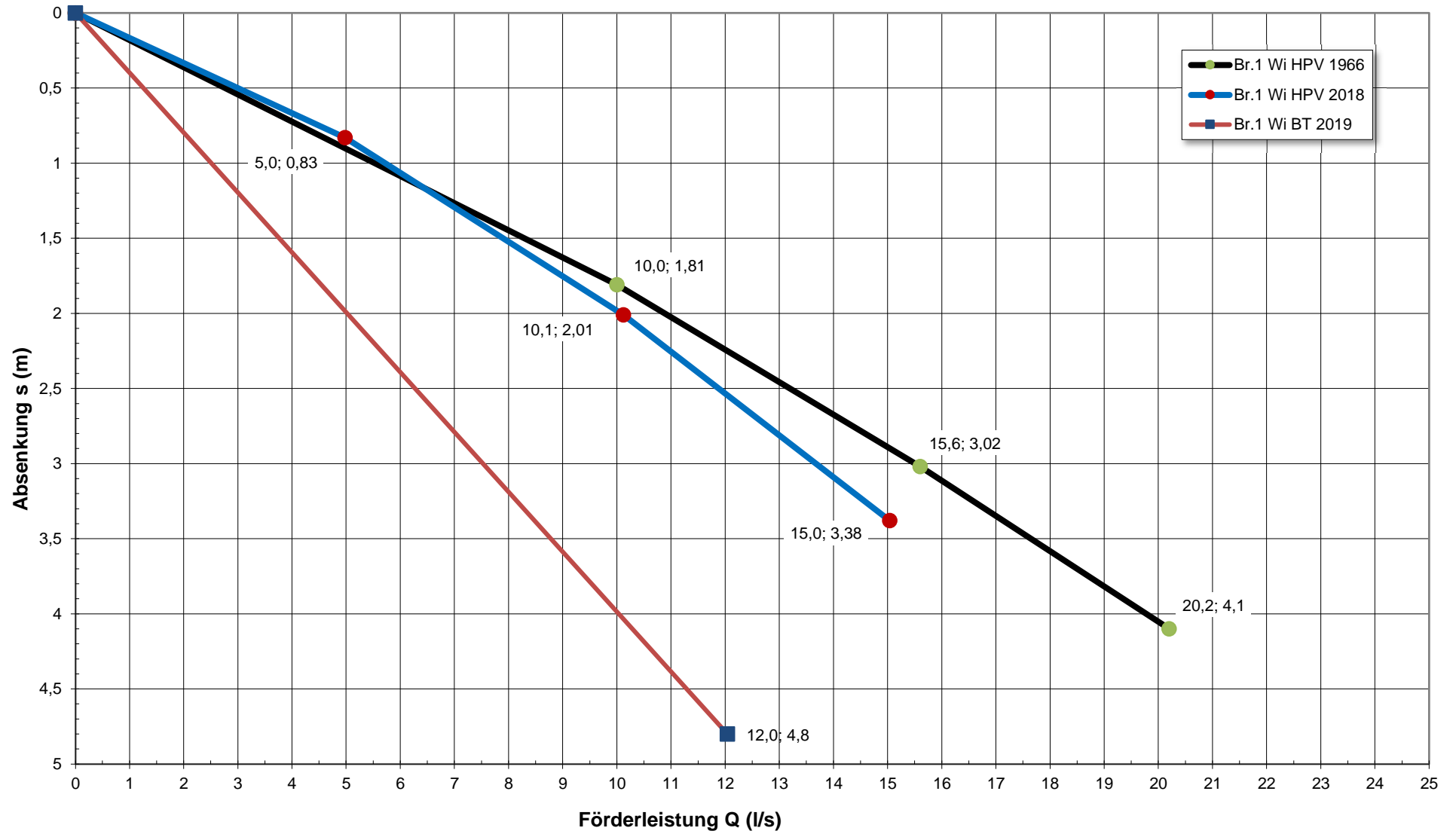
Q-s Diagramm: Brunnen 1 HPV 1966 (rückgebaut) / Brunnen 1 HPV Januar 2018 / Brunnen 1 BT März 2019
